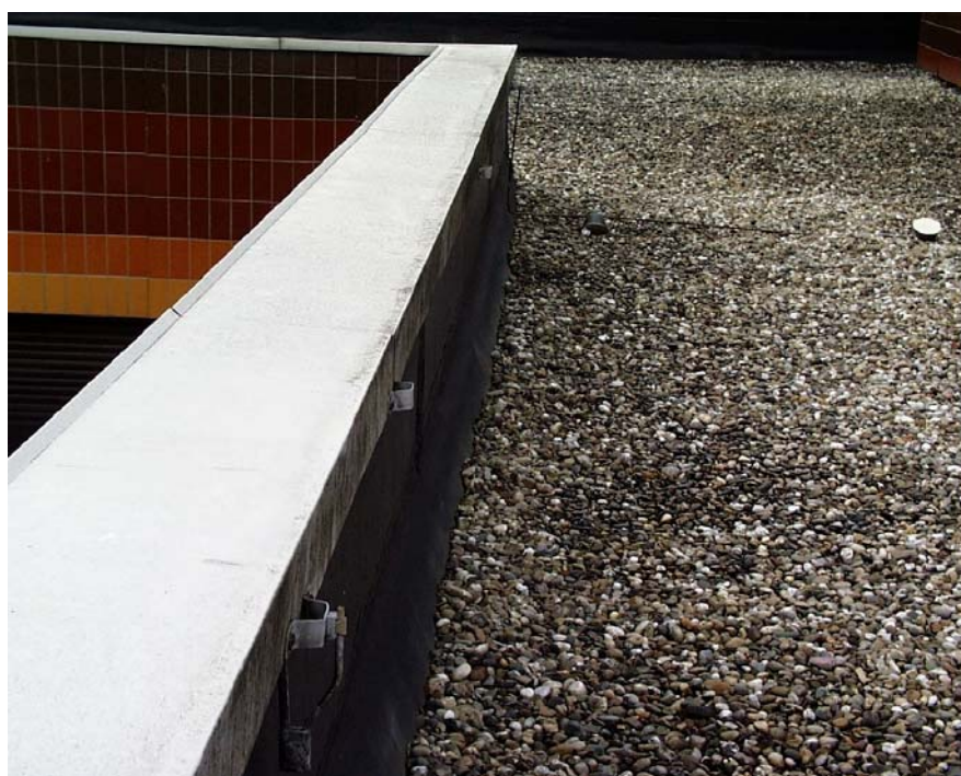
Bild 5: Übersichtsaufnahme der Attika des Objektes Berufsbildungszentrum Wadern nach 30 Jahren Liegezeit; keine Schrumpfspannungen erkennbar
